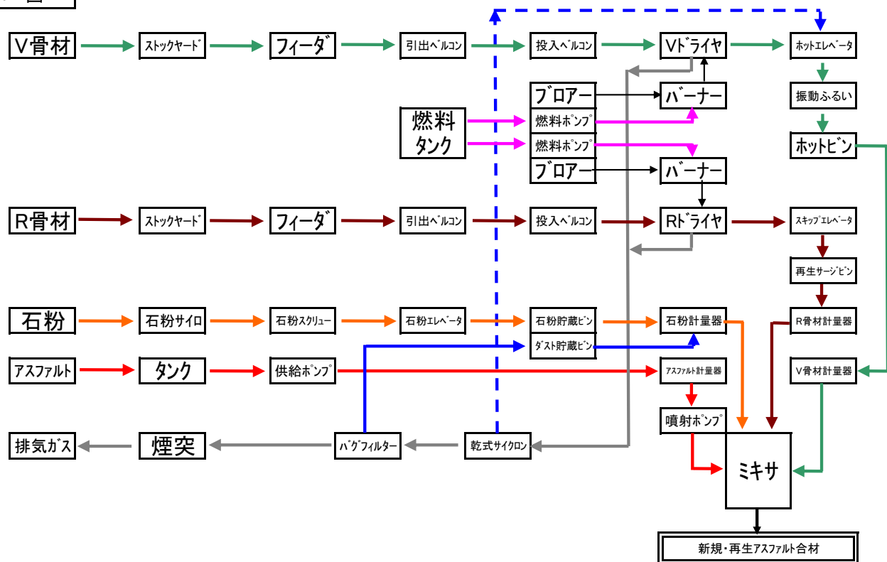
フロー図
